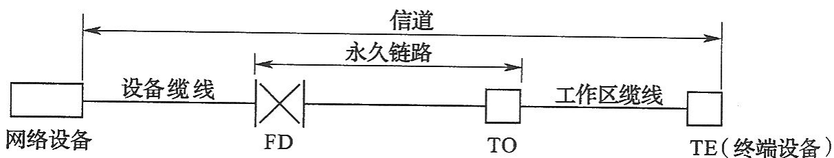
图 4 两个连接器件的信道与永久链路
